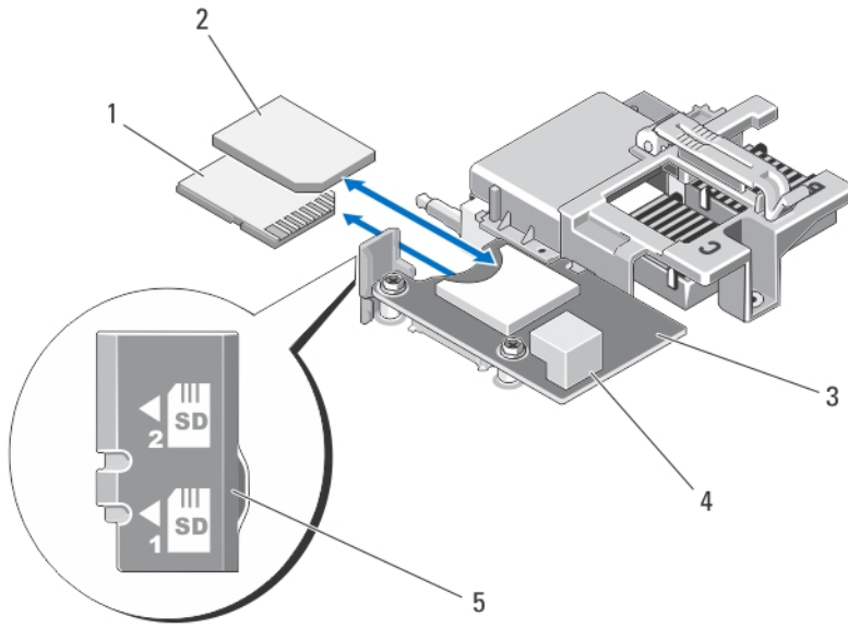
图 12: 更换 SD 卡
