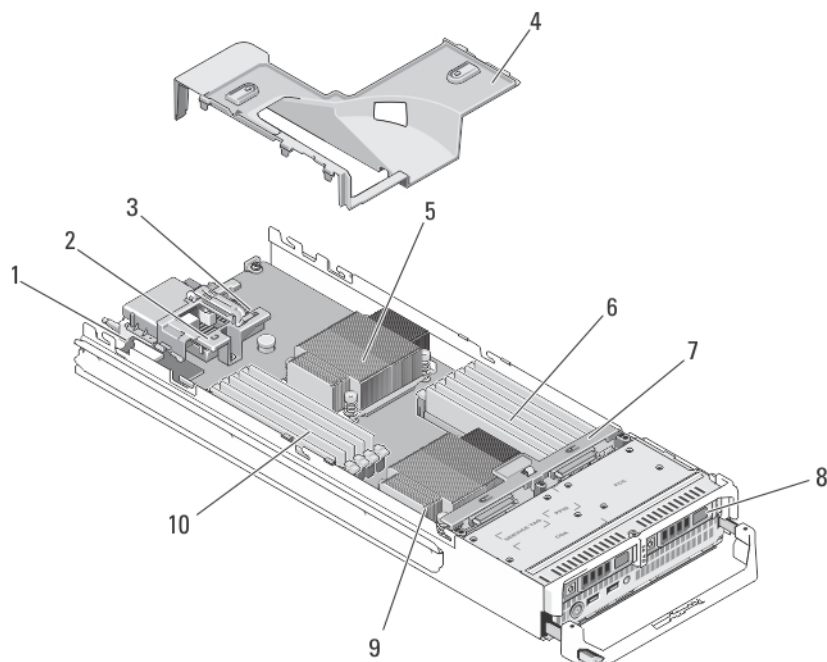
图 7: 服务器模块内部
