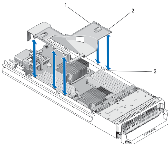
图 8: 卸下和安装冷却导流罩
