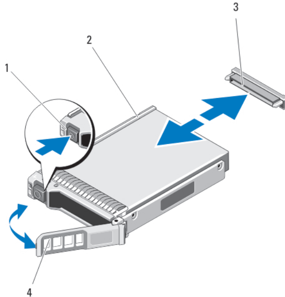
图 17: 卸下和安装硬盘驱动器/SSD
