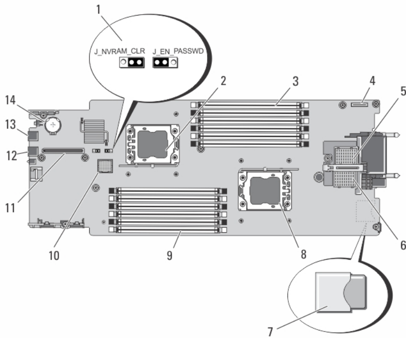
图 23: 系统板连接器
