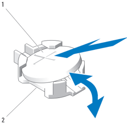
图 21: 更换 NVRAM 备用电池
