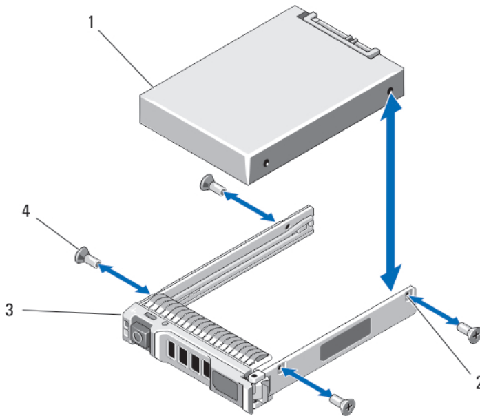
图 18: 在硬盘驱动器/SSD 托盘中卸下和安装硬盘驱动器/SSD
