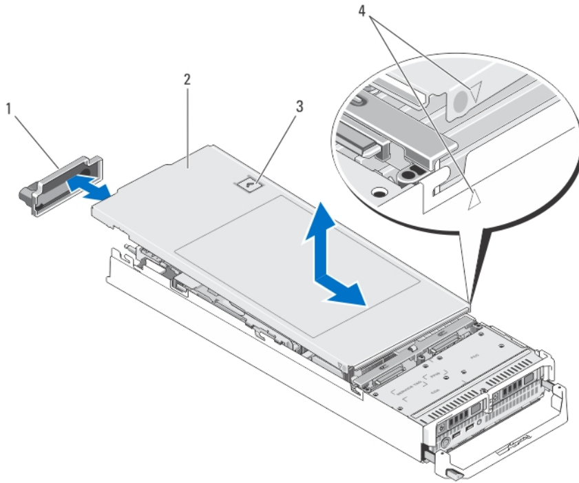
图 6: 打开与合上服务器模块
