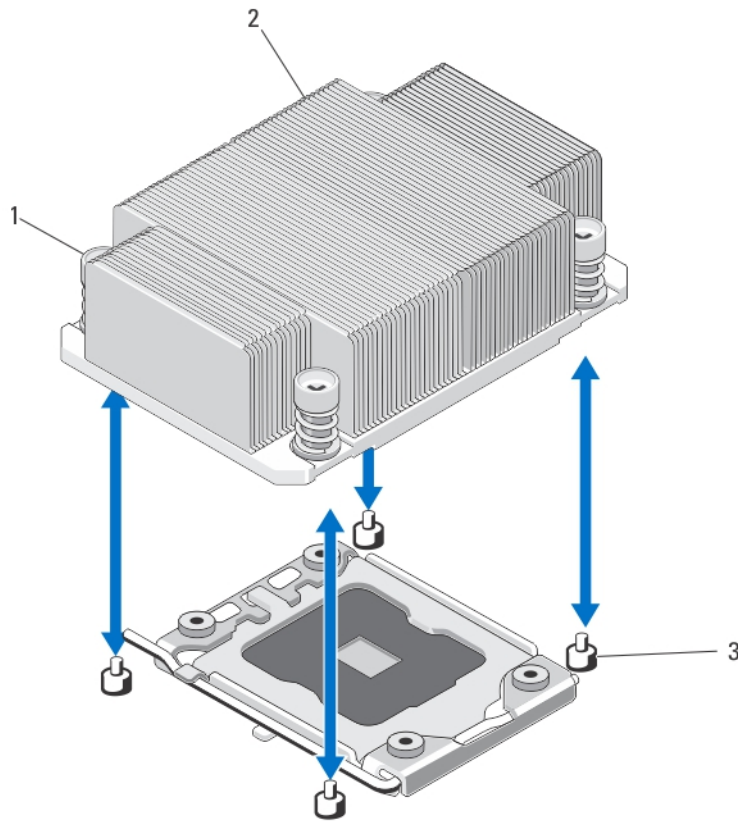
图 15: 卸下和安装散热器
