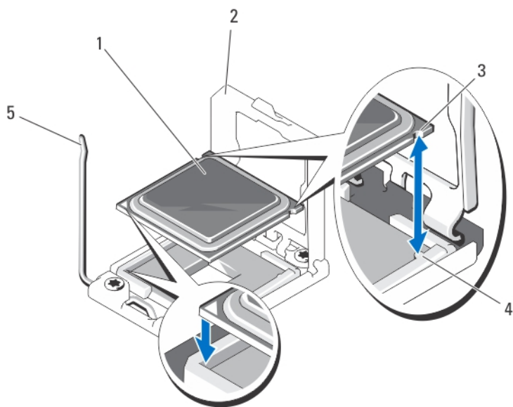
图 16: 卸下和安装处理器
